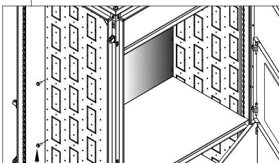
M6x16 Flanged hex head (11Nm) M6x16 Testa esagonale flangiata (11Nm)
