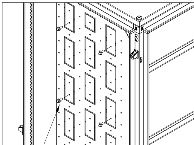
M6x16 Flanged hex head (11Nm) M6x16 Testa esagonale flangiata (11Nm)
