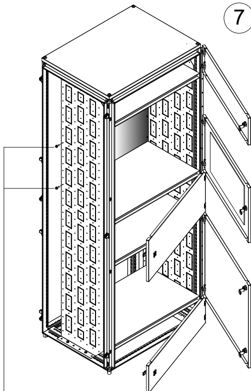
M6x16 Flanged hex head (11Nm) M6x16 Testa esagonale flangiata (11Nm)
